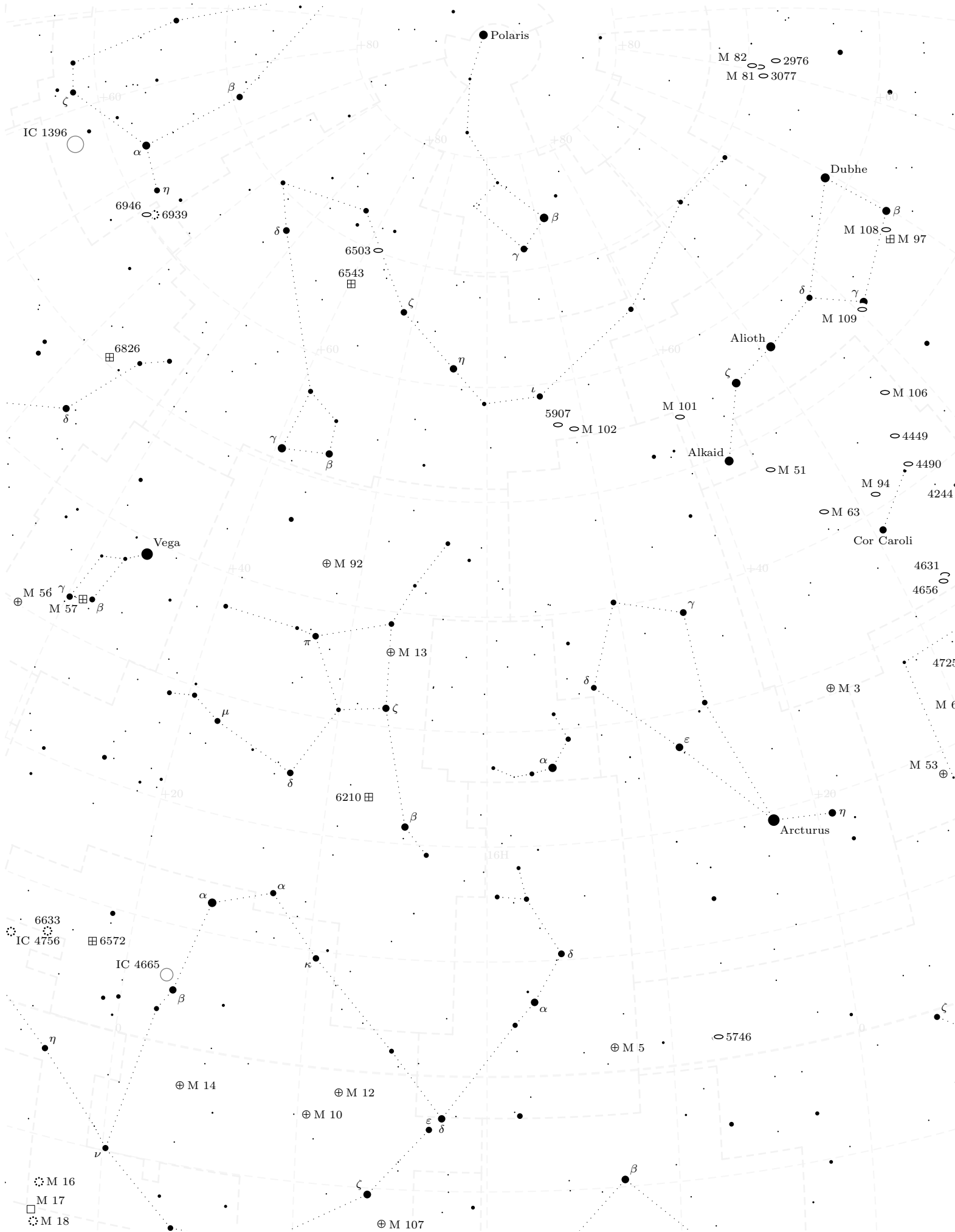
Chart 5: R.A. 16 h, Decl. +40 deg
